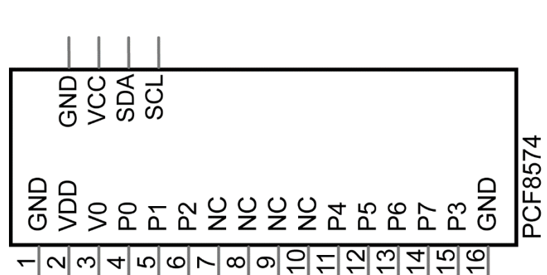
PCF8574 module pin diagram
