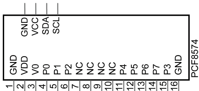
PCF8574 module pin diagram
